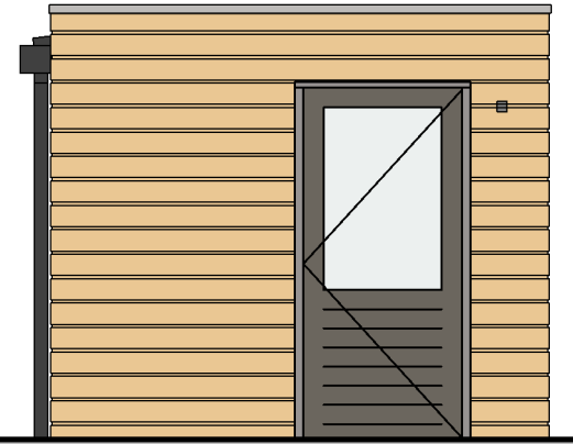
Linkergevel
